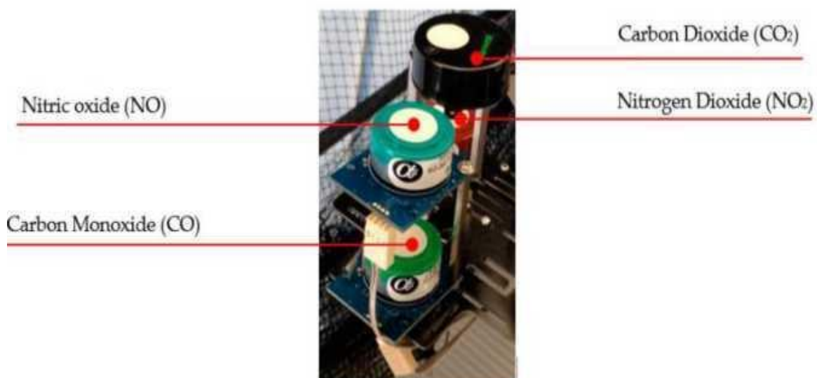
Obrázok 2: Dron s namontovanými senzormi na analýzu znečistenia ovzdušia.
