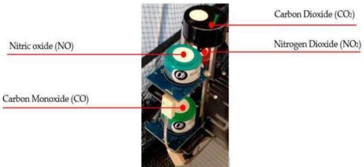
Rycina 3. Czujniki zanieczyszczenia powietrza które mogą być montowane do dronu.
