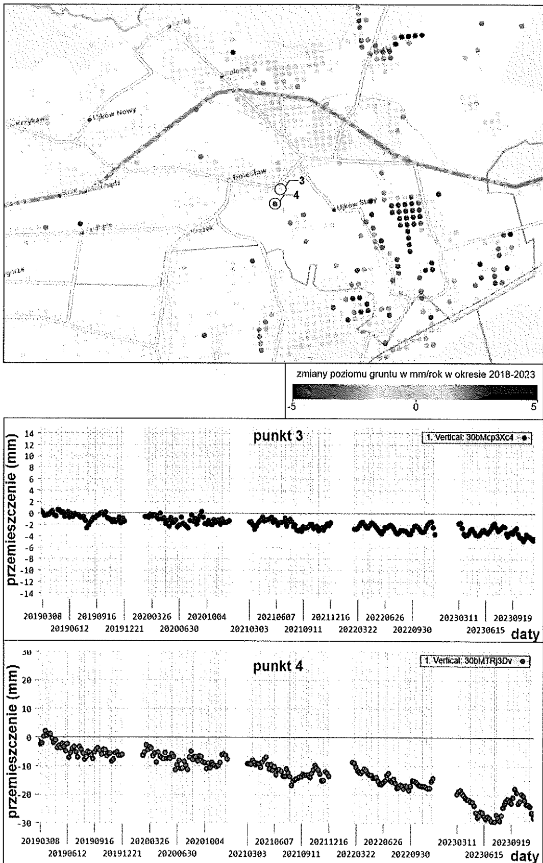
Rycina 4. Punkty w których, zobrazowano zmiany powierzchni gruntu wynikające ze zmian zwierciadła wody podziemnej w granicach 5 mm/rok (mapa u góry ryciny), oraz przebieg zmian powierzchni gruntu w wybranych punktach 3 i 4, w okresie 2019-2023.
