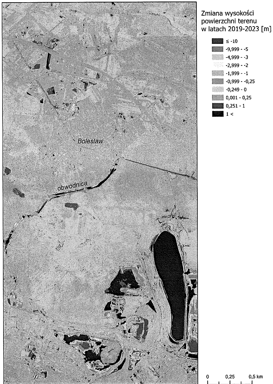
Rycina 7. Zmiany poziomu gruntu występujące w latach 2019-2023 na podstawie modeli terenu LiDAR
