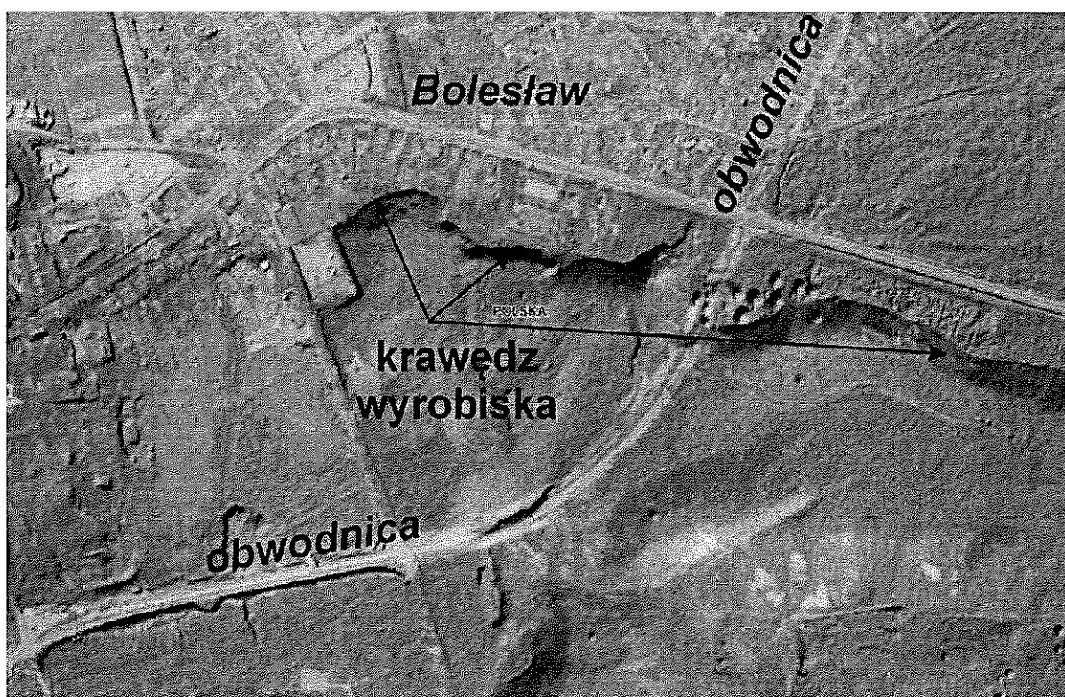
Rycina 5. Model terenu utworzony z danych LiDAR na podkładzie z ortofotomapy z widocznym przebiegiem obwodnicy Bolesławia oraz krawędziami wyrobiska.
