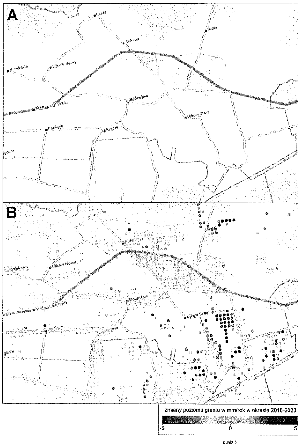
Rycina 1. Położenie badanego obszaru (A) oraz punkty, w których zobrazowano zmiany powierzchni gruntu wynikające ze zmian zwierciadła wody podziemnej w granicach 5 mm/rok (B).
